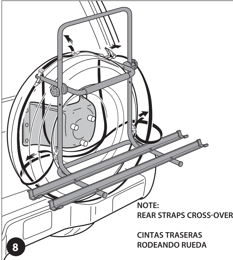
RUOTA A DESTRA SPARE WHEEL RIGHT RUEDA A LA DERECHA
